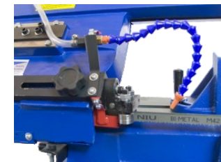
Sägeblattkühlung
