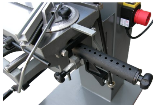
Dübelbohrereinrichtung
